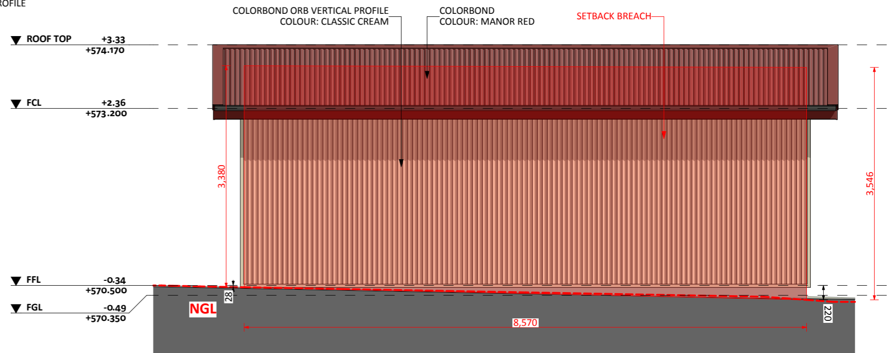
ELEVATION 04
