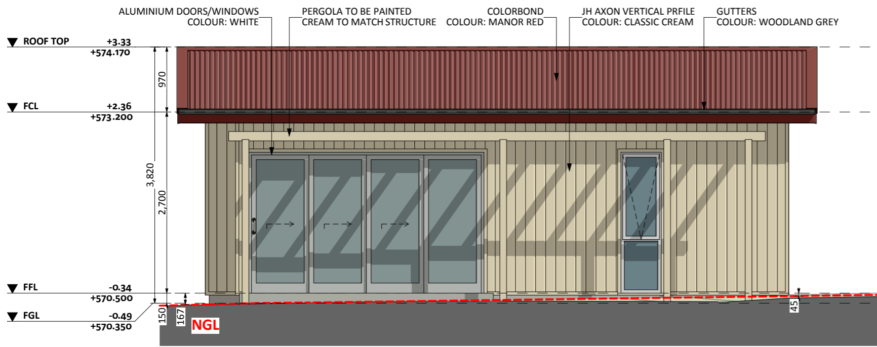
ELEVATION 01
