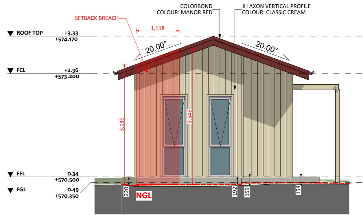
ELEVATION 02
