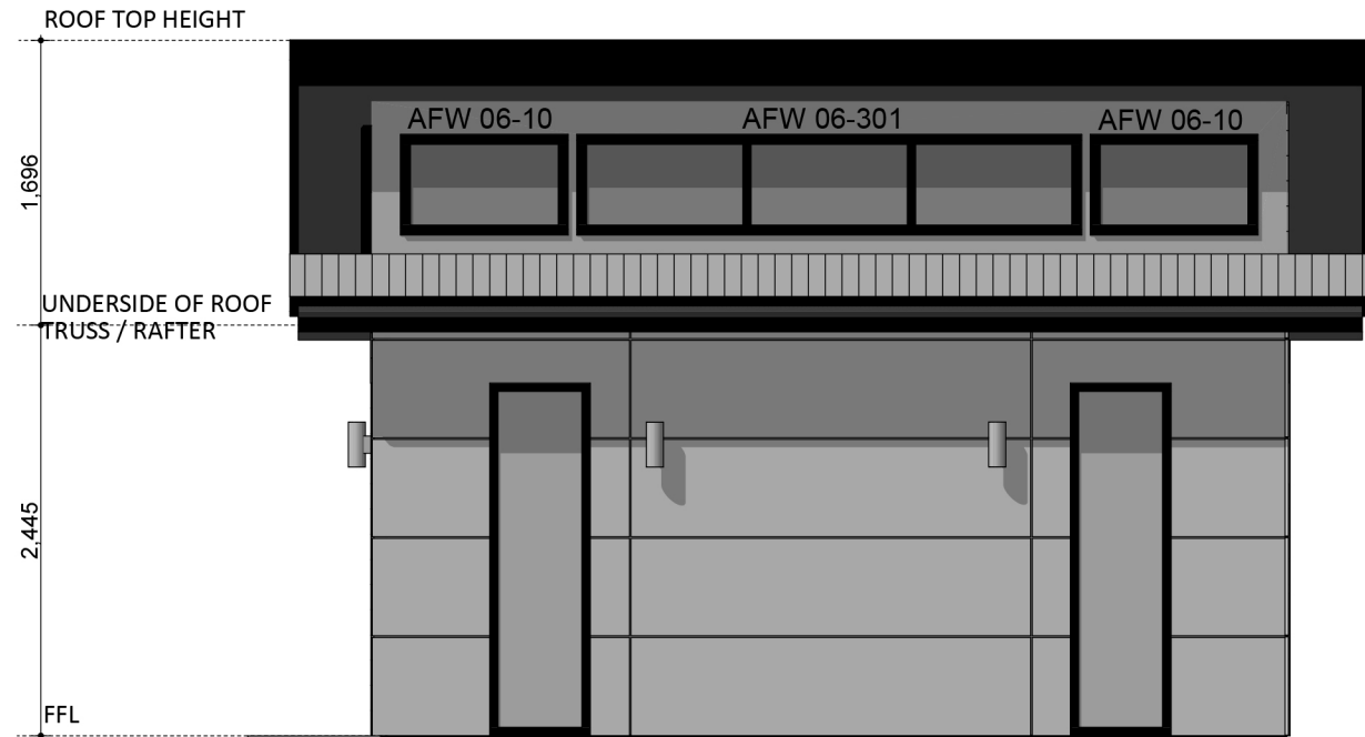
ELEVATION 02
