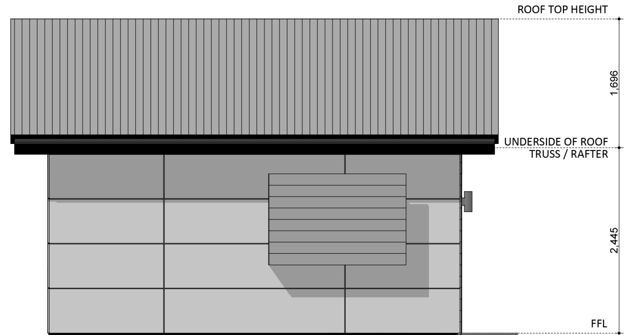
ELEVATION 04
