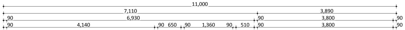
▽ ELEVATION 01
