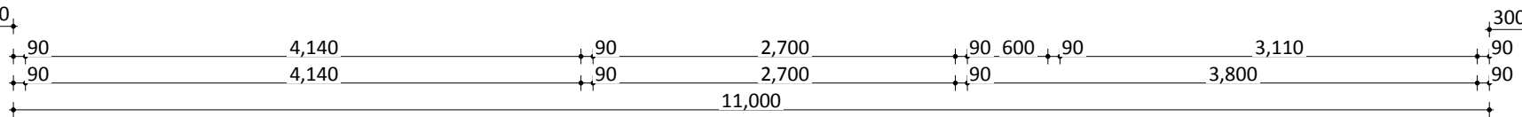
△ ELEVATION 03
