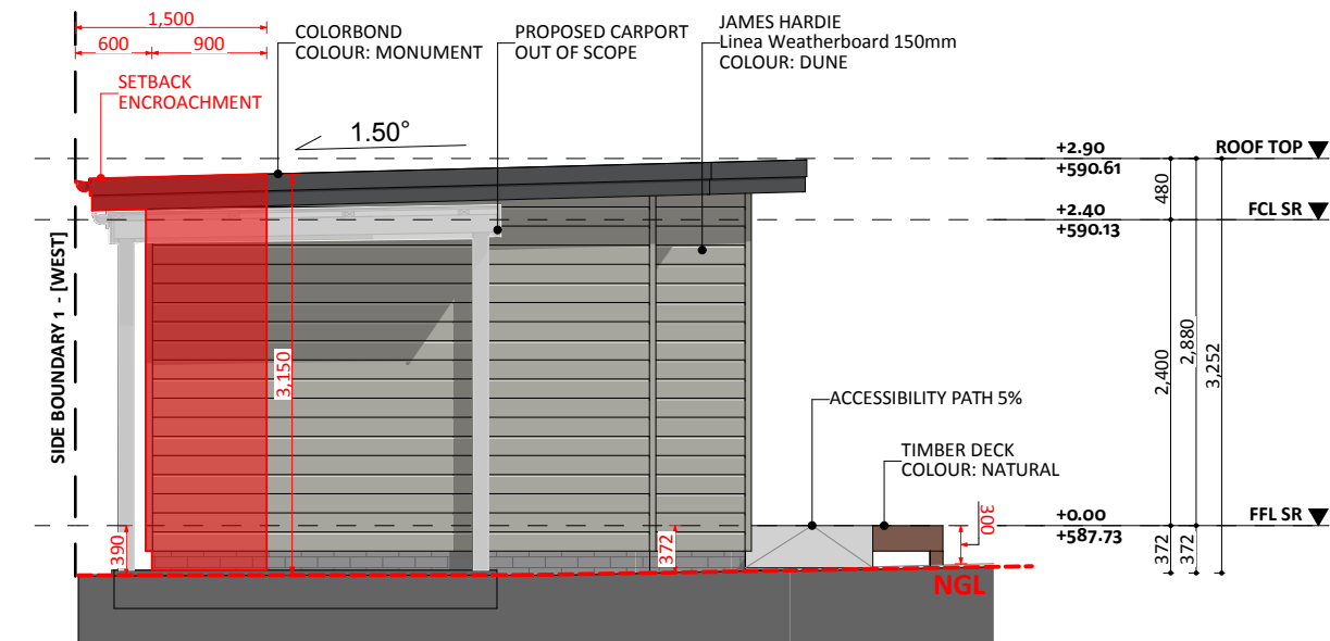
ELEVATION 04
