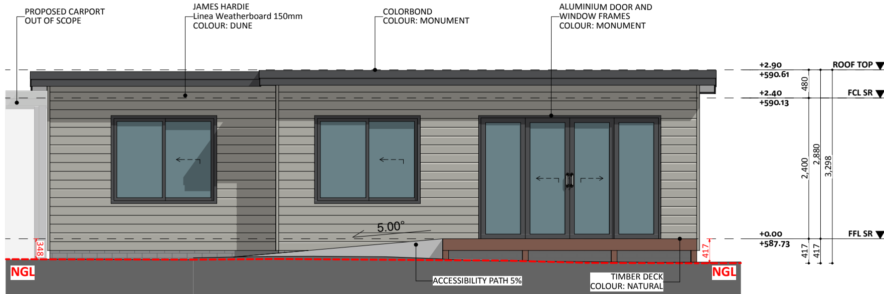
ELEVATION 01
